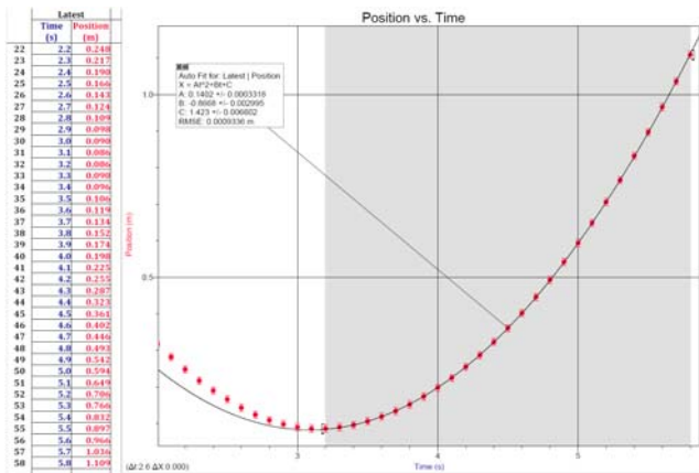
Σχήμα 2: Καταγραφίσεις πειραματικές τιμές της απόστασης αμαξιδίου-αισθητήρα συναρτήσει του χρόνου. Η προσαρμοσμένη καμπύλη στα δεδομένα του επιταχυνόμενου μέρους της κίνησης είναι πολυωνυμική δευτέρου βαθμού
