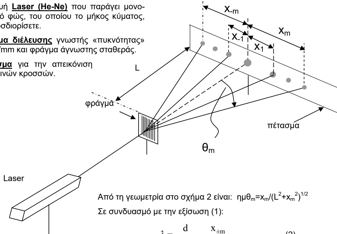
Σχήμα 2: Πειραματική διάταξη
