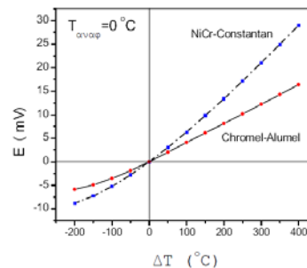
Σχήμα 2: Καμπύλη βαθμονόμησης των συνηθισμένων θερμοστοιχείων NiCr-Constantane και Chromel-Alumel.
