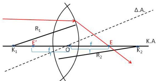
Σχήμα 1. Συγκλίνων φακός
