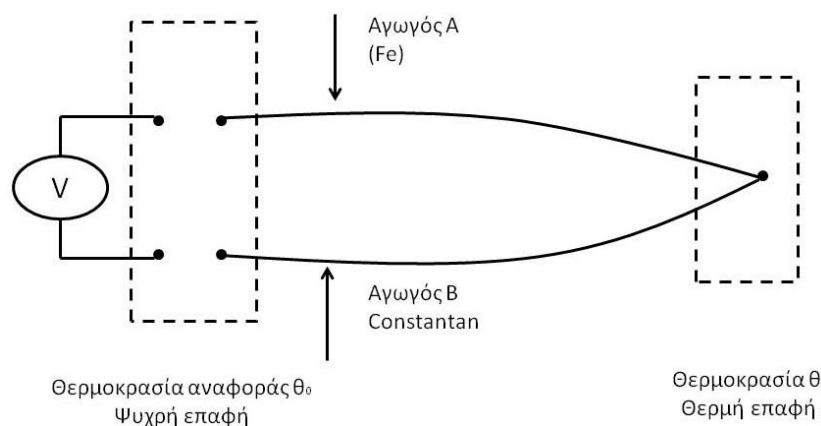
Σχήμα 1: Θερμοζεύγος
