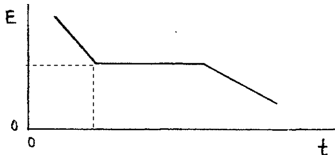
Σχήμα 4. Μεταβολή της θερμοκρασίας με το χρόνο κατά την πήξη του Sn
