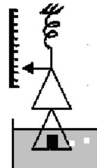
Σχήμα 1: Ζυγός Jolly.
