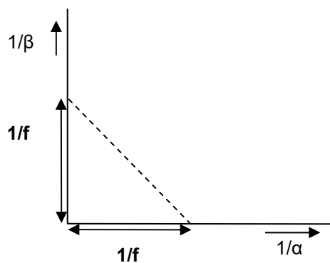
Σχήμα 3: Γραφική απεικόνιση της συνάρτησης 1/\beta = \varphi(1/\alpha)
