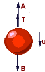
Σχήμα 1: Δυνάμεις που ασκούνται σε σφαίρα που κινείται με ταχύτητα u μέσα σε υγρό.
