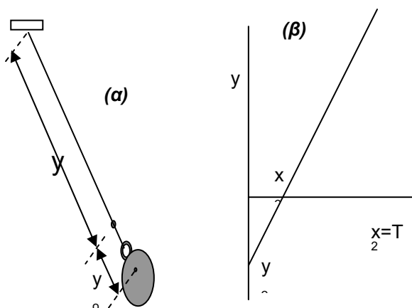
Σχήμα 1: (α) Ορισμός των μηκών y και y_0 . (β) Η ευθεία y=(g/4\pi^2)x-y_0 έχει κλίση K=\Delta y/\Delta x=g/4\pi^2 και συντεταγμένες επί την αρχή: x_0=(4\pi^2/g)y_0 και -y_0 .
