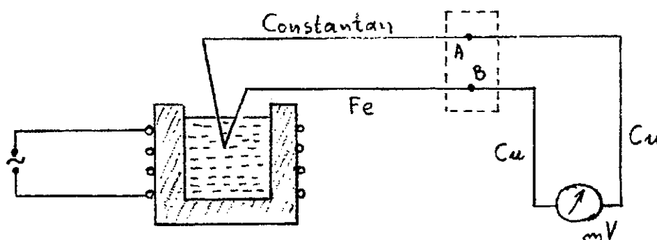
Σχήμα 3. Πειραματική διάταξη
