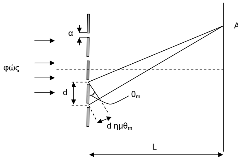
Σχήμα 1: Σχηματική παράσταση οπτικού φράγματος διέλευσης και σχηματισμού κροσσών συμβολής σε πέτασμα.
