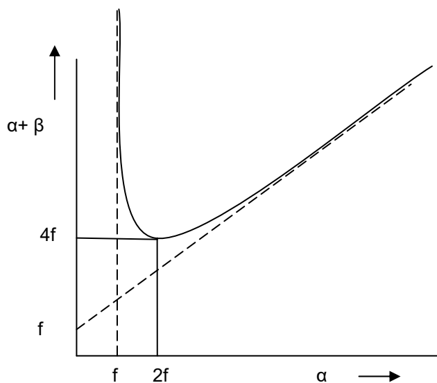
Σχήμα 4: Γραφική απεικόνιση της συνάρτησης \alpha + \beta = g(\alpha) .
